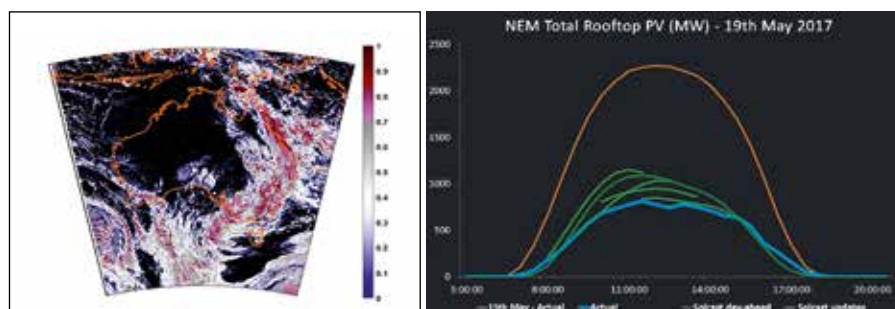
Obrázek č. 4: Mraky mohou v australské soustavě znamenat mezidenní změnu výkonu i o 1000 MW. Zdroj: Jo Nova
